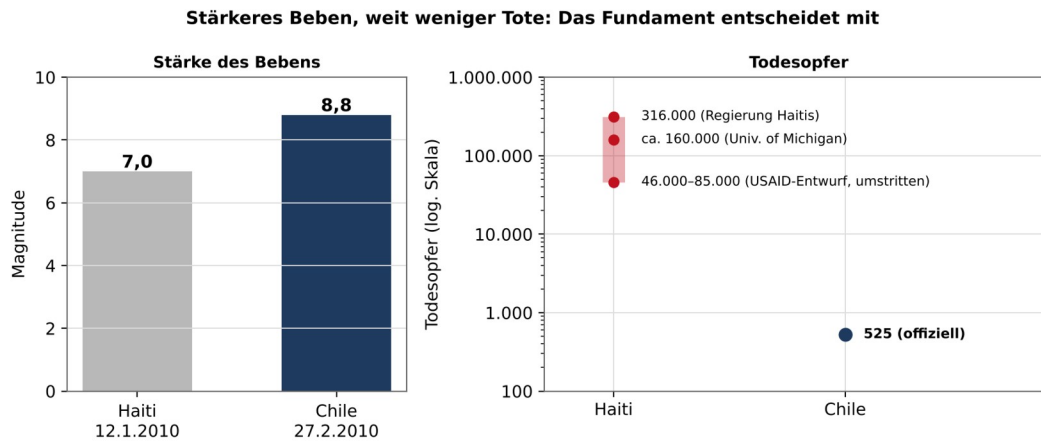
Abb. 16: Zwei Erdbeben, zwei Fundamente – Stärke und Todesopfer der Beben in Haiti und Chile 2010. Todesopfer logarithmisch, für Haiti die Spanne der Schätzungen. Datenquellen: Wikipedia nach USGS, Regierung Haitis, University of Michigan; Regierung Chiles; NPR.
